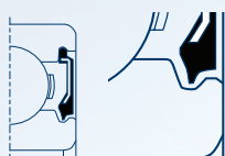
LLB T°: -25°C / +120°C
