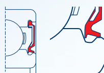
LLU T°: -25°C / +120°C
