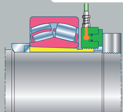
Bucha de aperto
