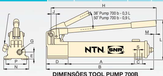
DIMENSÕES TOOL PUMP 700B
