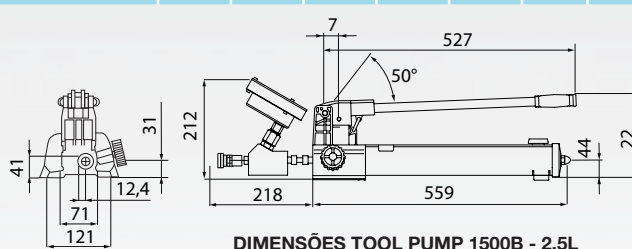
DIMENSÕES TOOL PUMP 1500B - 2,5L
