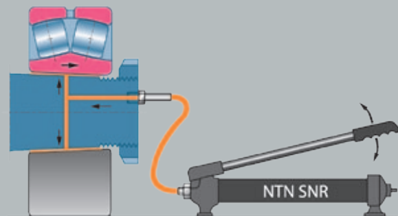
Eixos com suporte cônico
