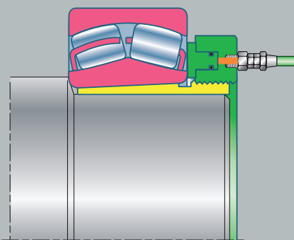
Bucha de desmontagem
